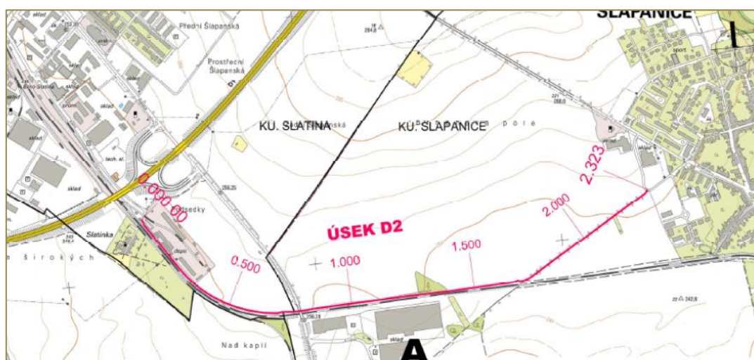
Přehledová situace 1. etapy – cyklostezky Šlapanicko (řešené úseky jsou vyznačeny růžovou barvou, vč. označení úseku) – pokračování viz níže přehledky jednotlivých úseků
